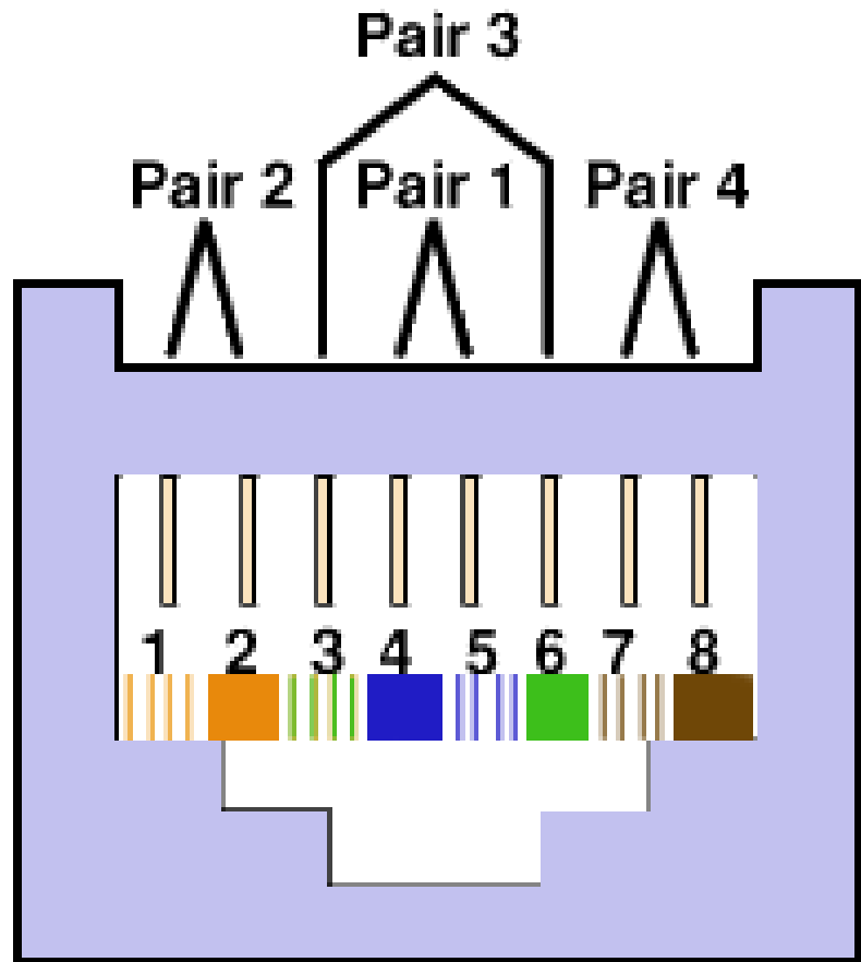
T568B
