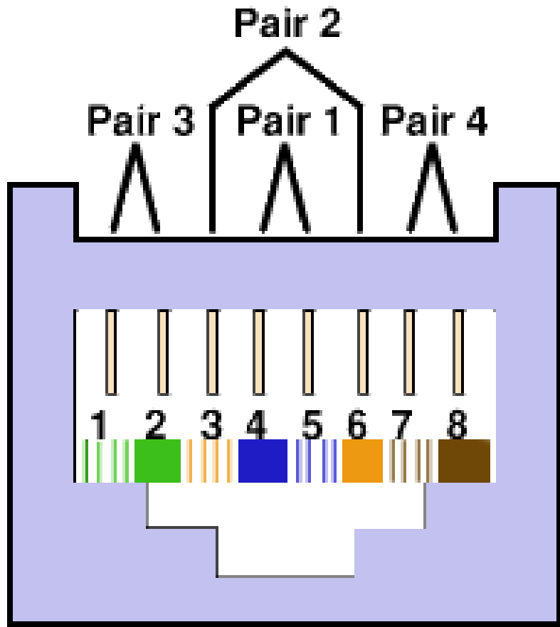
T568A
